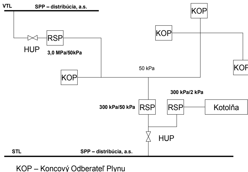
Schéma lokálnej distribučnej siete LDS – BA - Kopčianska
