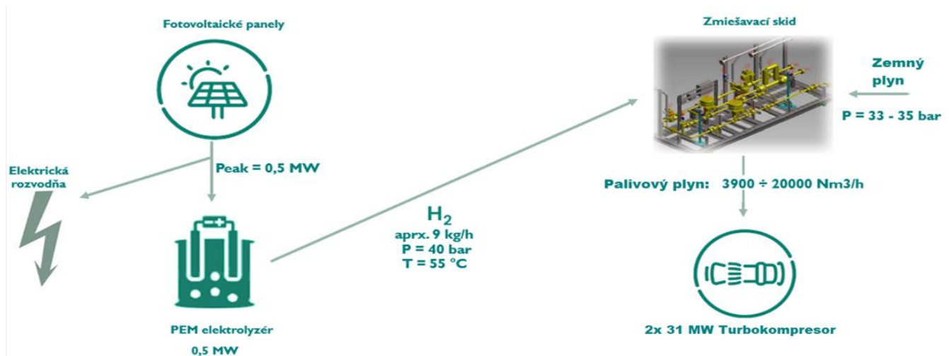
Obrázok č. 5 - schéma Green H2 na KS01
