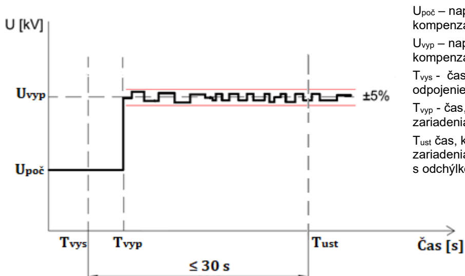
Obr. F9.6.9 Skúška automatického odpojenia kompenzačného zariadenia
