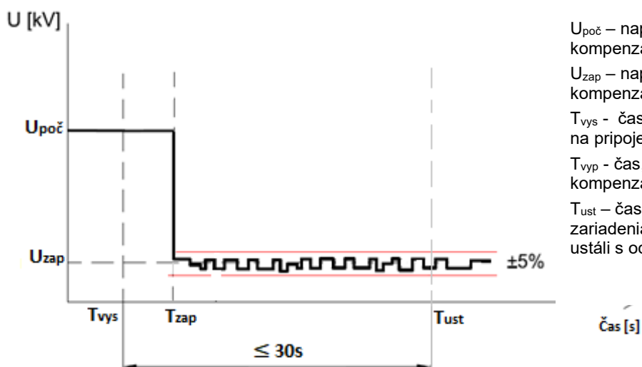
Obr. F9.6.10 Skúška opätovného pripojenia kompenzačného zariadenia
