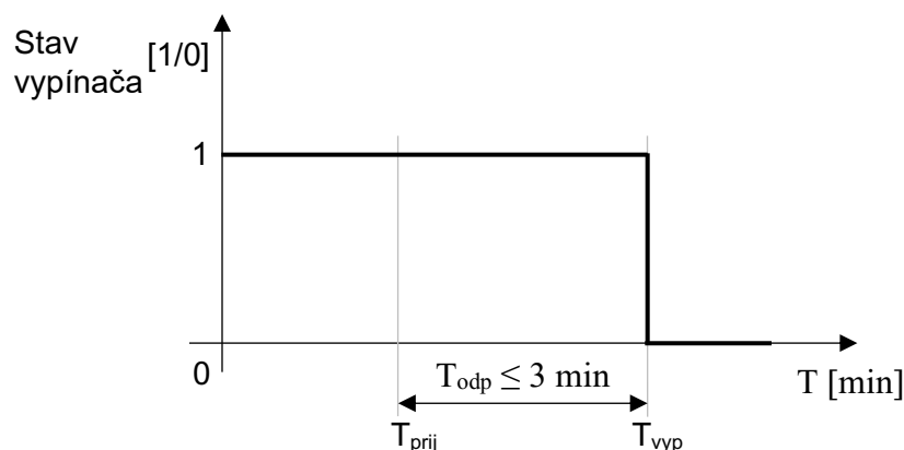
Obr. F9.6.5 Skúška odpojenia zariadenia
