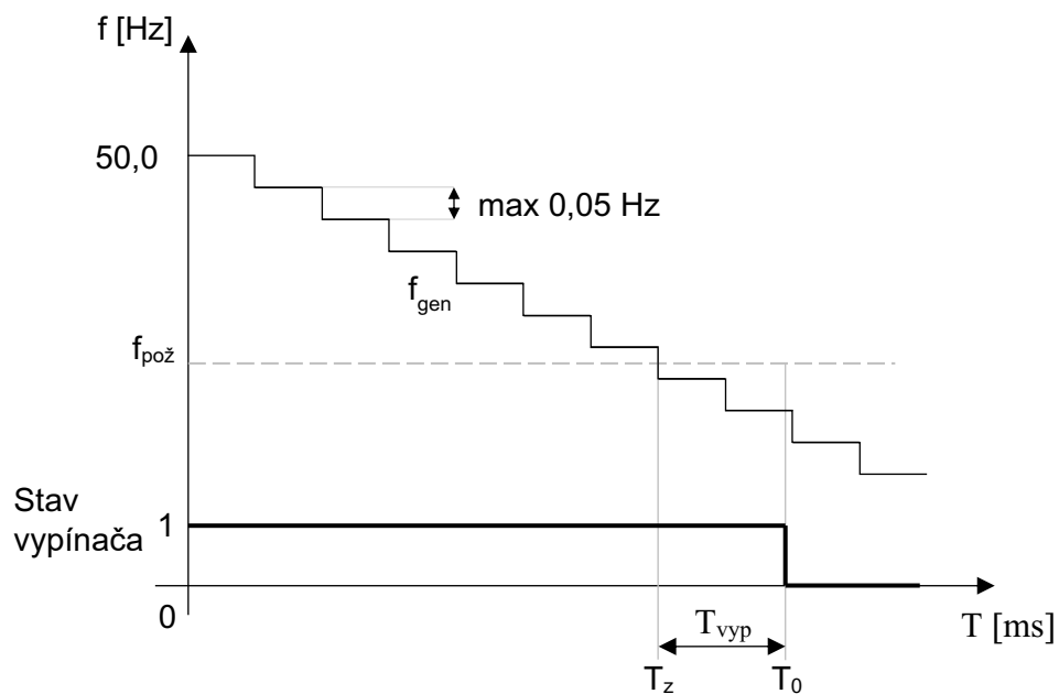
Obr. F9-6.1 Skúška frekvenčného odľahčenia
