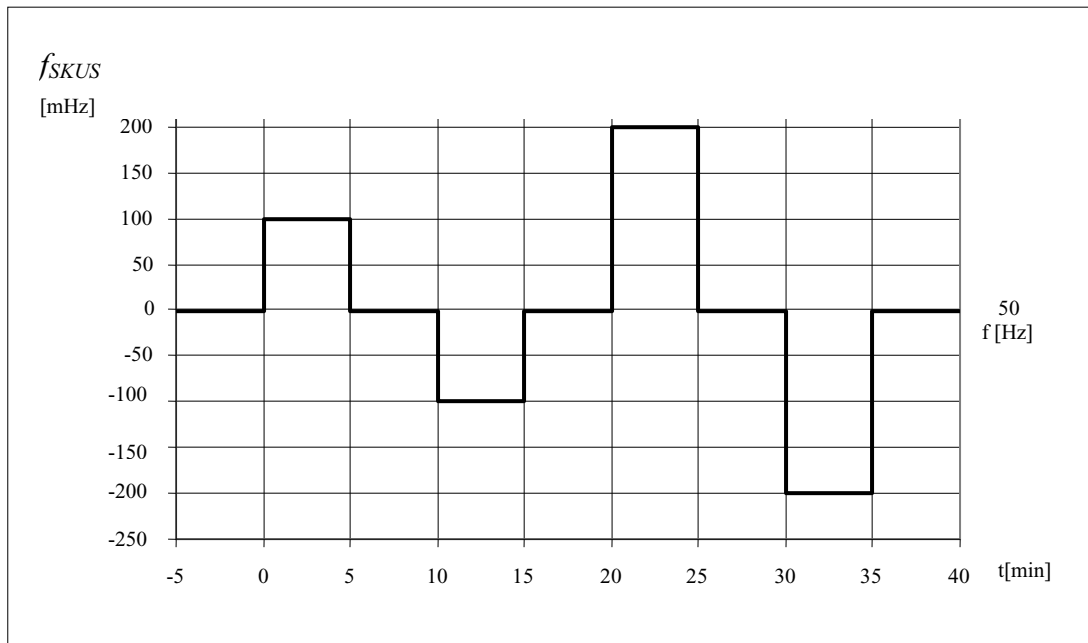
Obr. F1.1 Skúšobný signál pre overenie akčieschopnosti FCR
