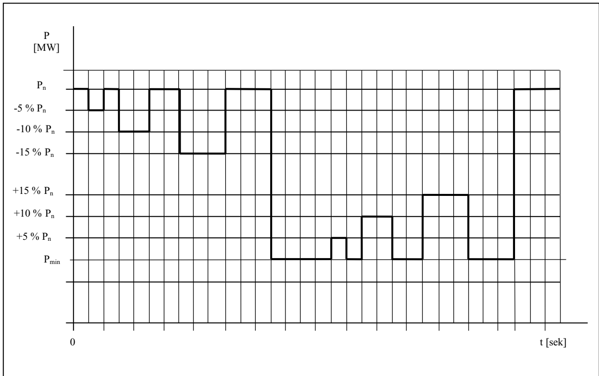
Obr. F1.2a Skúšobný signál pre overovanie aFRR+/aFRR-
