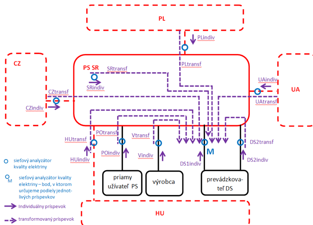
Obr. F75.1 Znáznornenie jednotlivých príspevkov od užívateľov PS daného kvalitatívneho ukazovateľa kvality elektriny v mieste „M“
