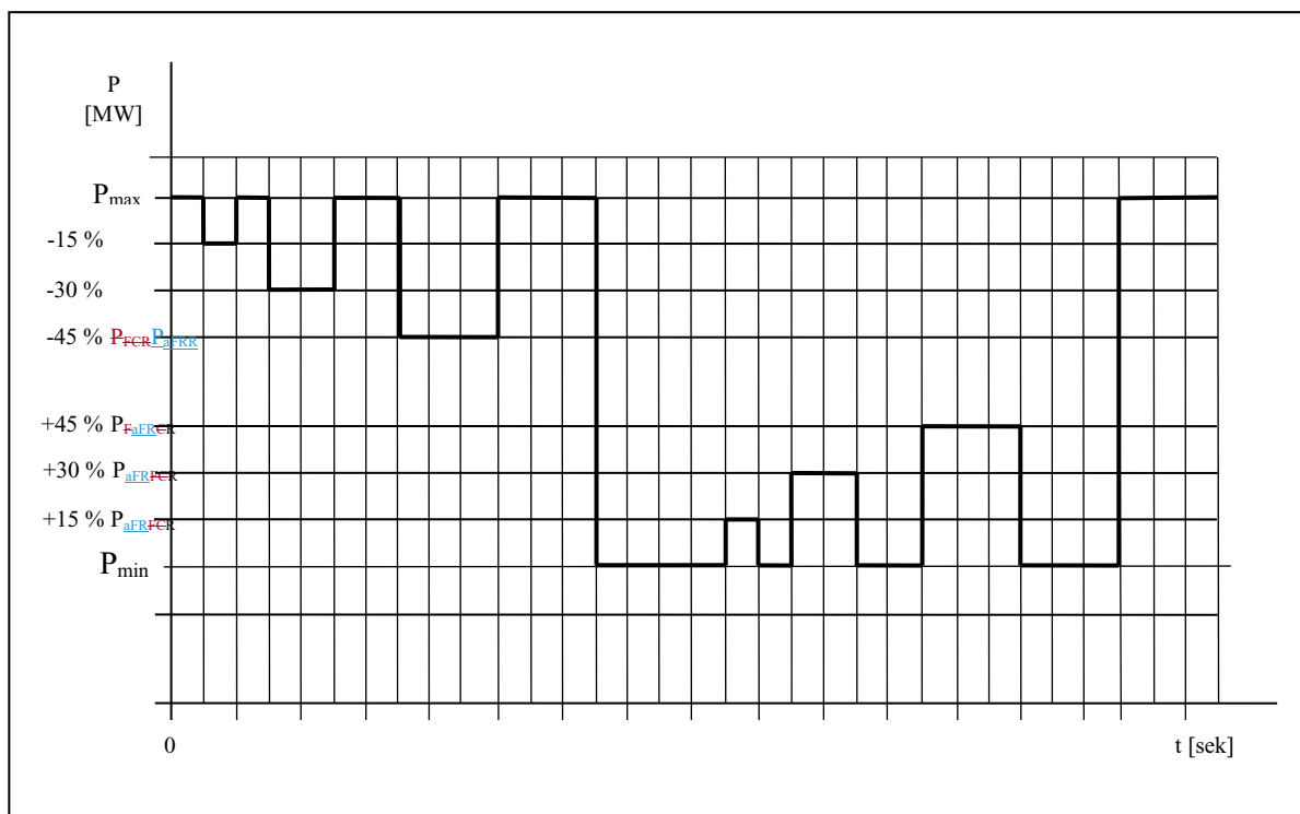
Obr. F1.2b Skúšobný signál pre overovanie aFRR+/aFRR-
