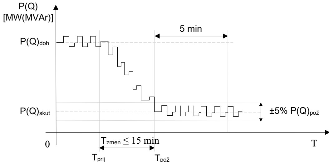
Obr. F9.6.8 Skúška zmeny odobraného výkonu
