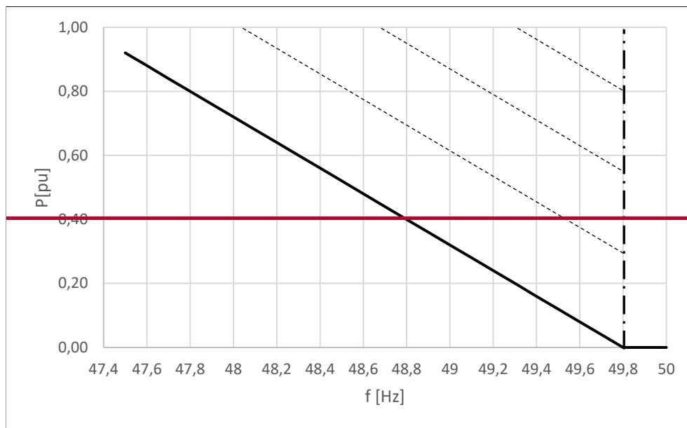
Obr. 6.2. Schopnosť odozvy činného výkonu na zmenu frekvencie zariadení na uskladňovanie elektriny
