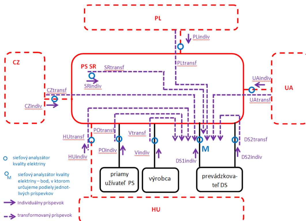
Obr. F7F5.1 Znázornenie jednotlivých príspevkov od užívateľov PS daného kvalitatívneho ukazovateľa kvality elektriny v mieste „M“
