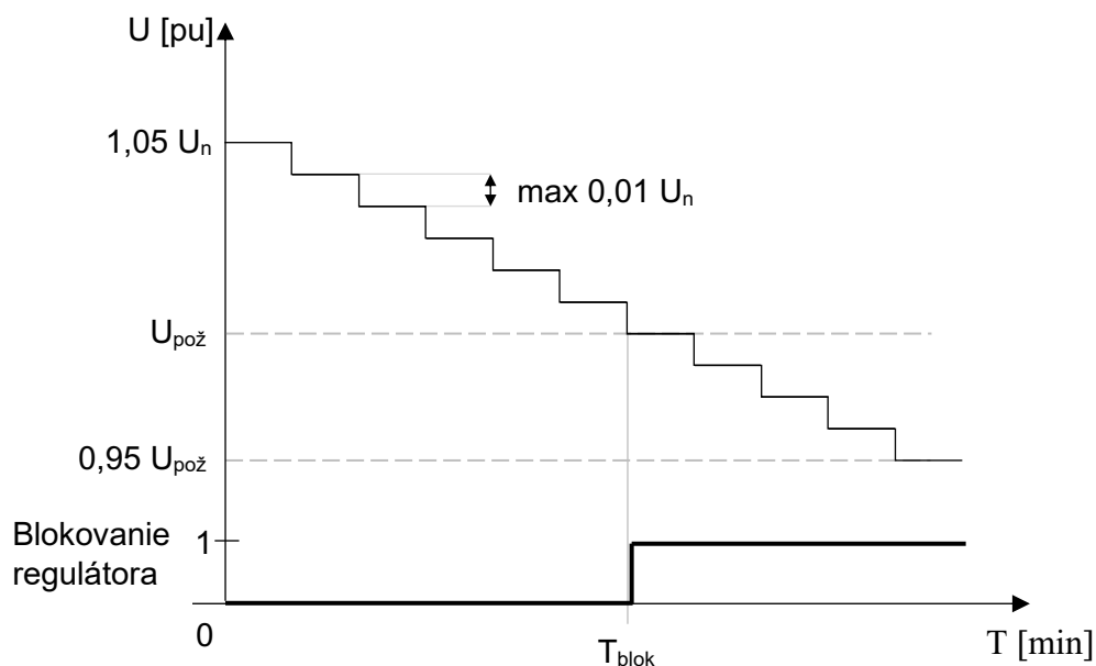
Obr. F9-6.6 Skúška blokovania prepínania odbočiek
