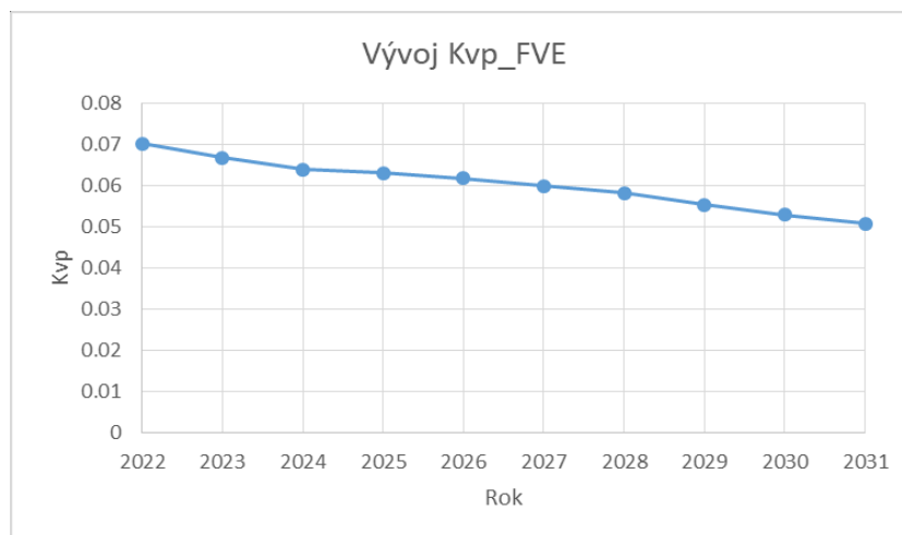
Obr. F43.2 Predpokladaný vývoj k_{vp} pre FVE
