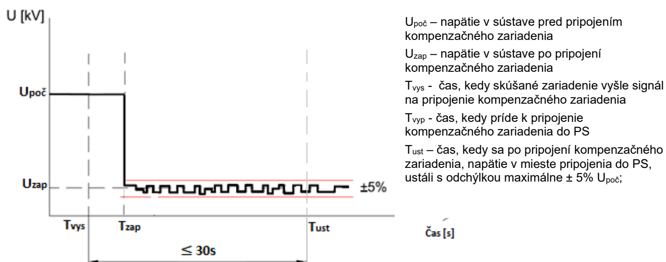
Obr. F9.6.10 Skúška opätovného pripojenia kompenzačného zariadenia
