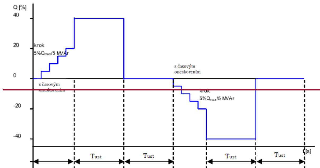
Obr. F8.13 Časový priebeh skúšobného signálu pre skokovú zmenu jalového výkonu
