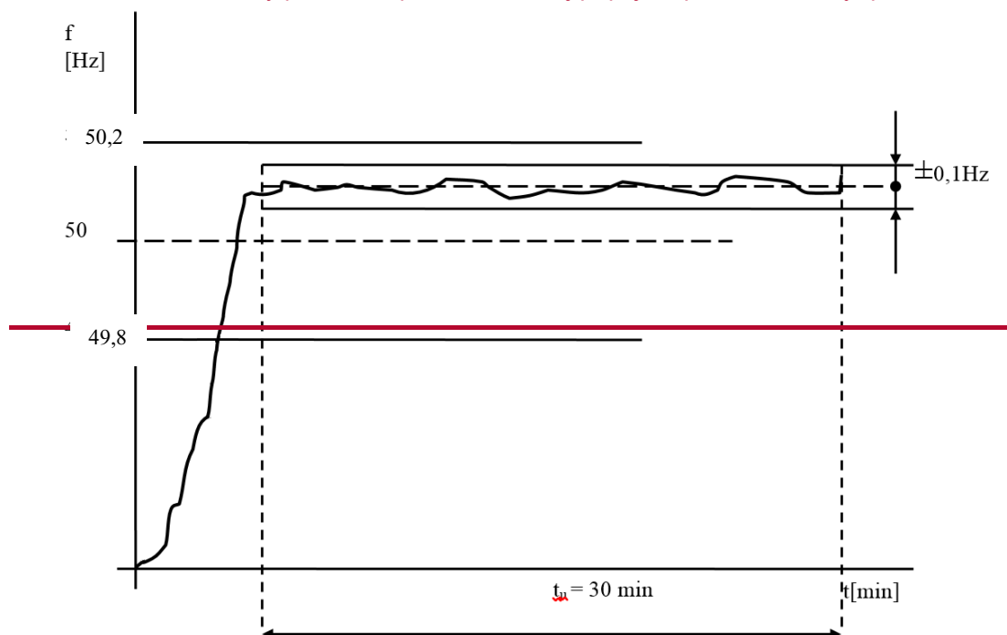
Obr. F1.4 Požadovaný priebeh frekvencie na určenej prípojnici pri "Štarte z tmy" pri ustálení
