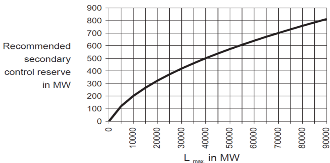
Obr. F43.1 Závislosť základnej zložky aFRR na L_{max}
