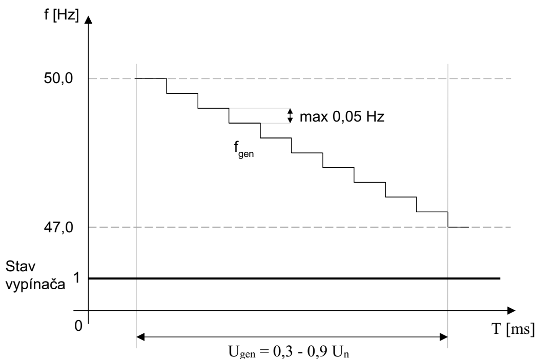
Obr. F9.6.2 Skúška blokovania frekvenčného odľahčenia
