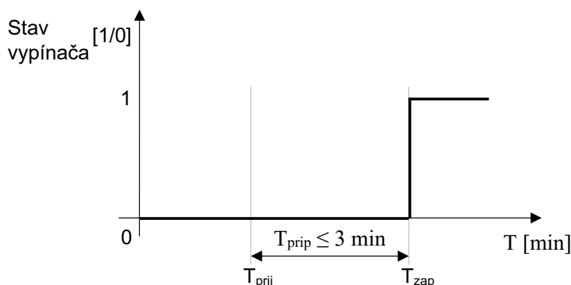
Obr. F9.6.7 Skúška opätovného pripojenia zariadenia
