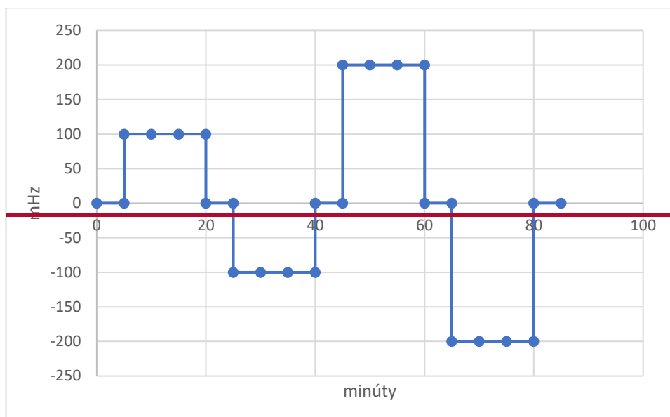
Obr. F 8.1 Skúšobný signál na overenie odozvy činného výkonu na zmenu frekvencie
