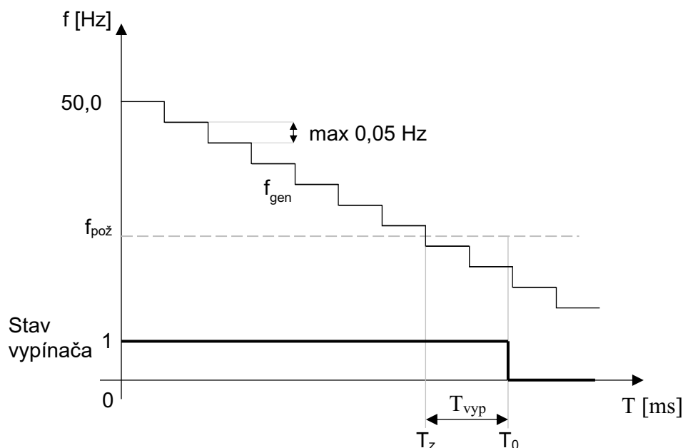
Obr. F9.6.3 Skúška frekvenčného odľahčenia
