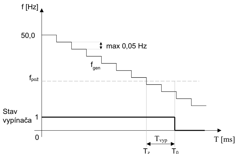
Obr. F9.6.1 Skúška frekvenčného odľahčenia
