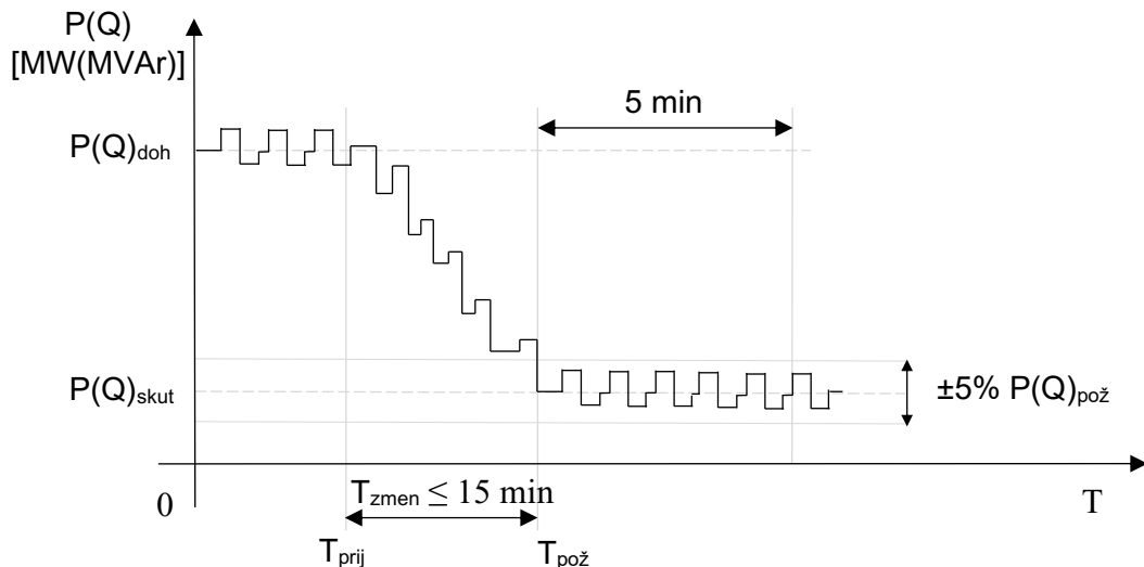
Obr. F9.6.8 Skúška zmeny odbraného výkonu
