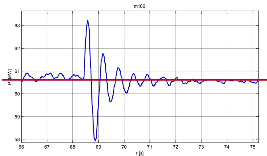
Obr. F1.6 Príklad prechodovej charakteristiky činného výkonu – skok hore – PSS zapnutý
