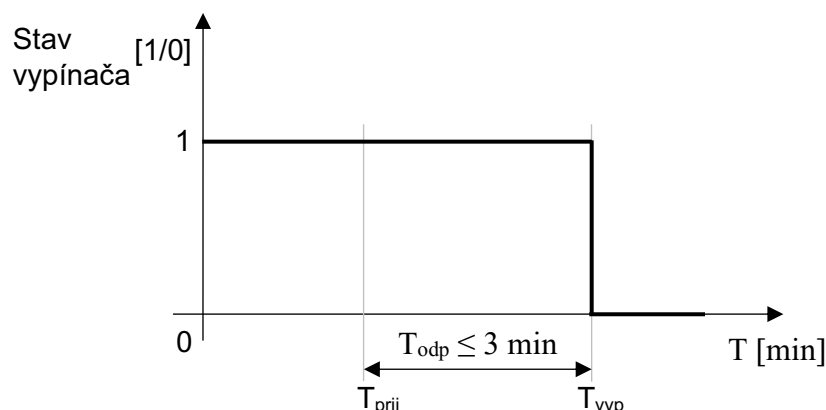
Obr. F9.6.5 Skúška odpojenia zariadenia
