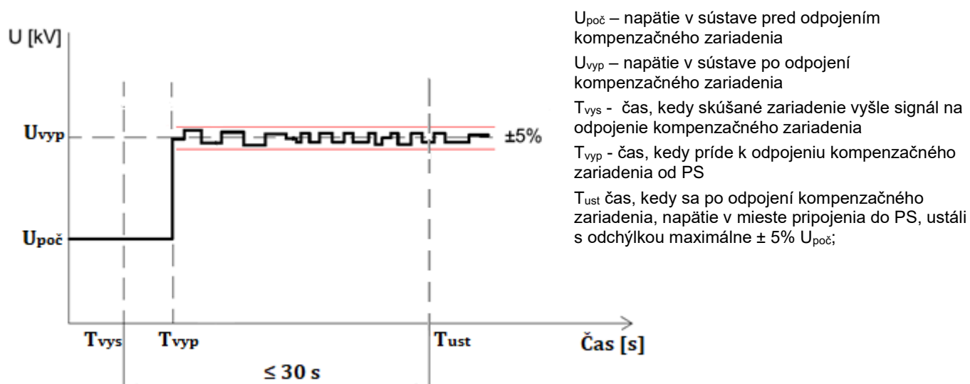
Obr. F9.6.9 Skúška automatického odpojenia kompenzačného zariadenia
