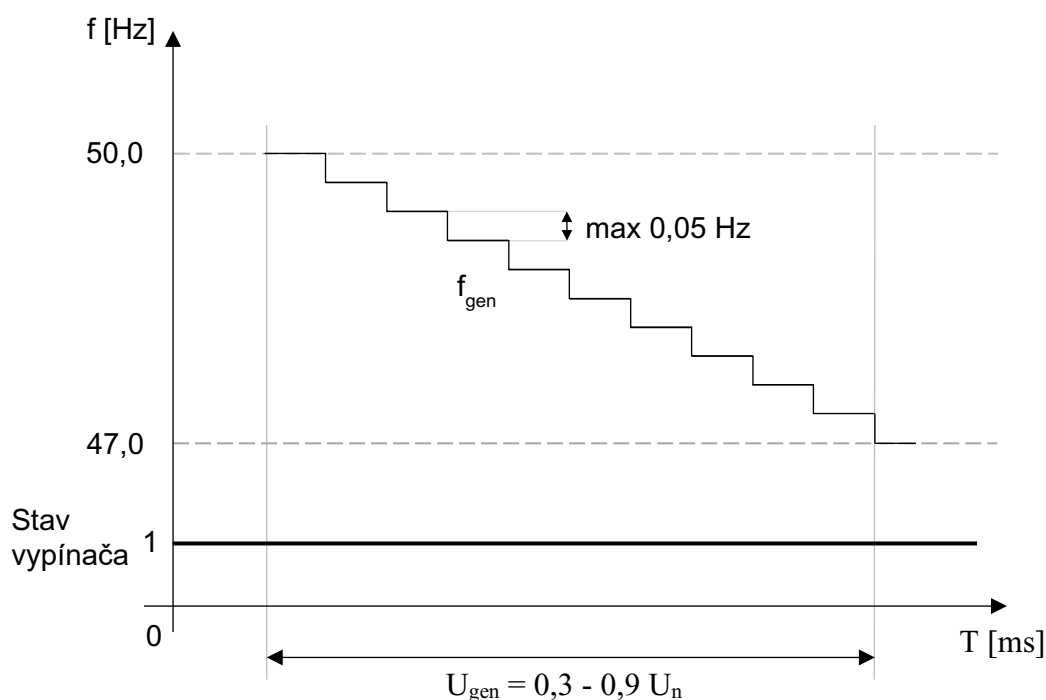
Obr. F9.6.4 Skúška blokovania frekvenčného odľahčenia
