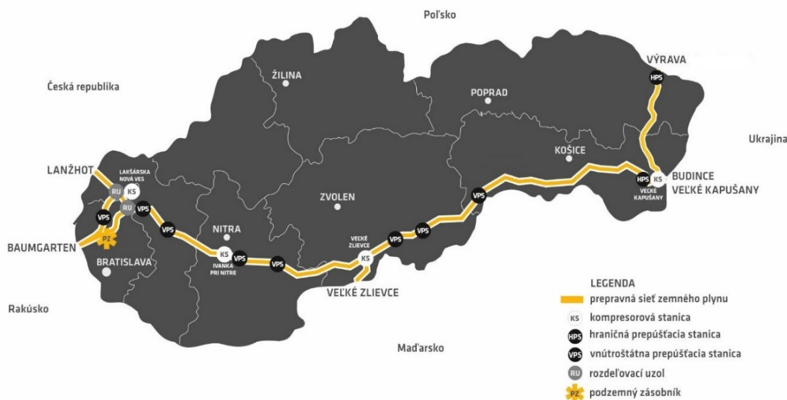
Obrázok č. 2: Prepravný systém prevádzkovaný spoločnosťou Eustream 4
