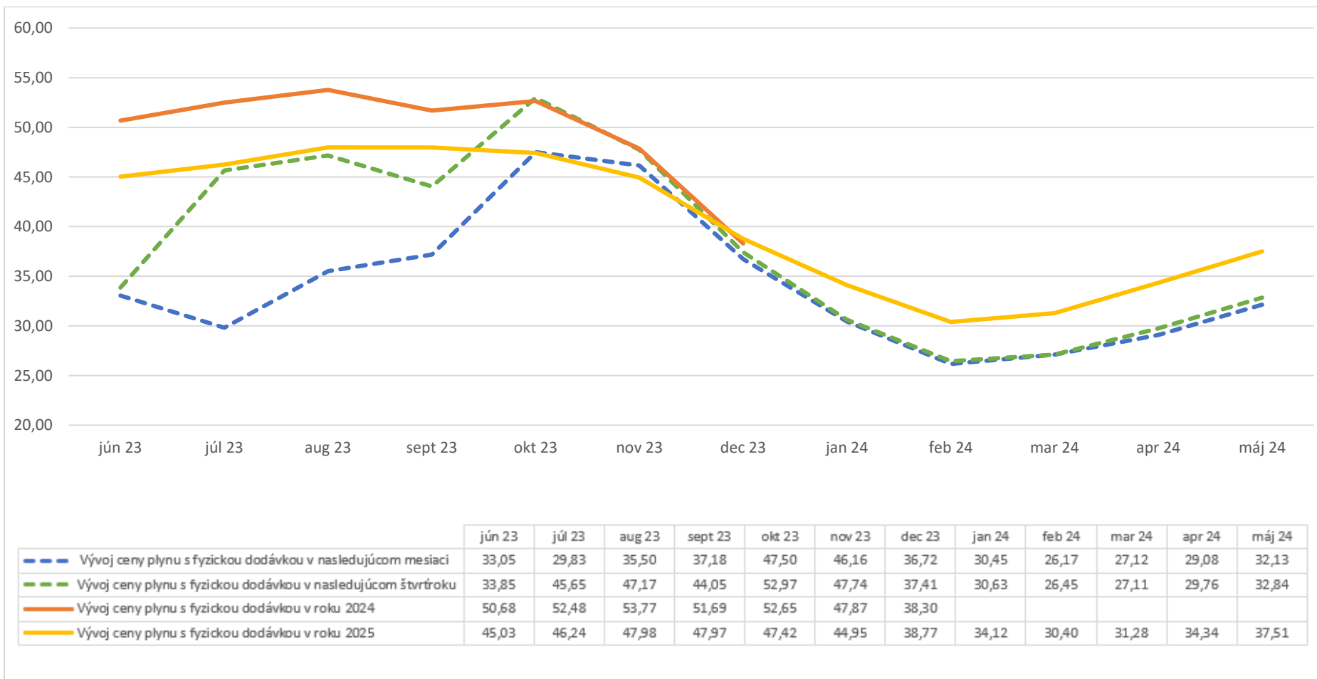
Graf č.3: Vývoj veľkoobchodných cenových indexov [EUR/MWh] plynu Trading Hub Europe EEX
