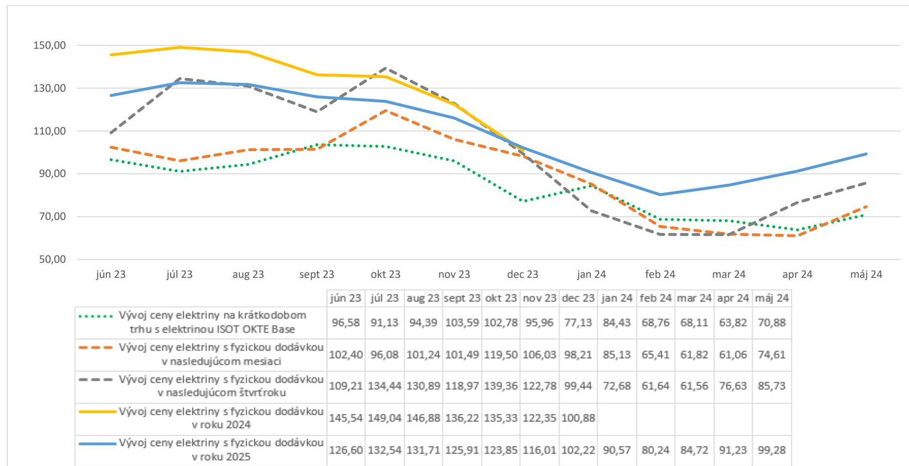
Graf č.1: Vývoj veľkoobchodných cenových indexov [EUR/MWh] elektriny PXE a OKTE
