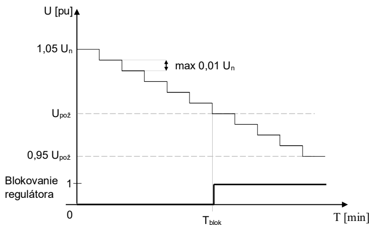
Obr. F6.6 Skúška blokovania prepínania odbočiek
