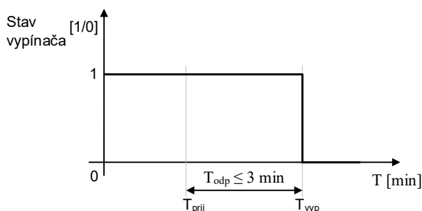
Obr. F6.5 Skúška odpojenia zariadenia
