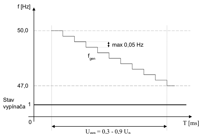
Obr. F6.4 Skúška blokovania frekvenčného odľahčenia
