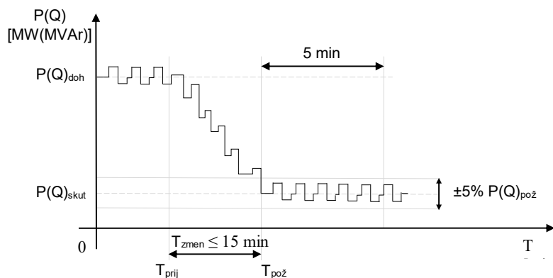
Obr. F6.8 Skúška zmeny odoberaného výkonu
