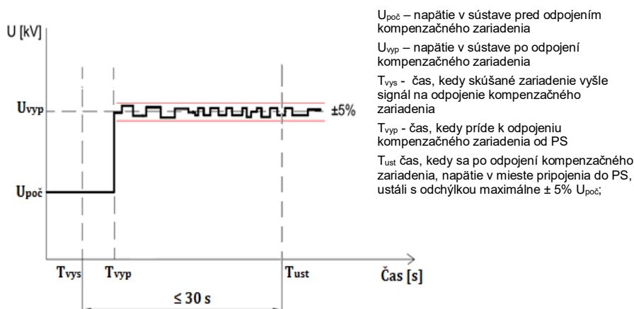
Obr. F6.9 Skúška automatického odpojenia kompenzačného zariadenia
