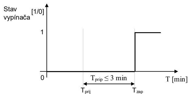
Obr. F6.7 Skúška opätovného pripojenia zariadenia
