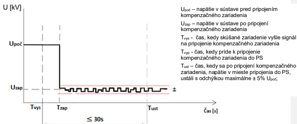
Obr. F6.10 Skúška opätovného pripojenia kompenzačného zariadenia
