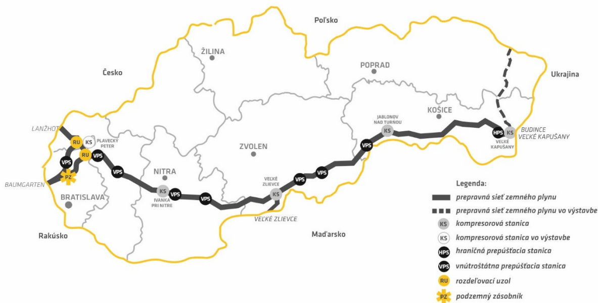
Obrázok č. 2: Prepravný systém prevádzkovaný spoločnosťou Eustream 1
