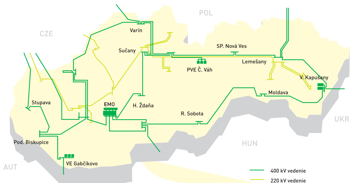
Prenosová sústava Slovenskej republiky
