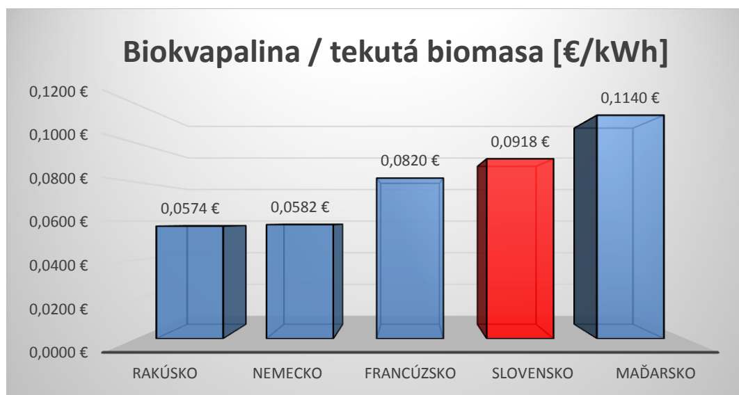
Graf 10: Grafické porovnanie hodnoty výkupnej ceny pre zariadenia využívajúce tekutú biomasu (Slovensko – kategória (E), (Rakúsko – tekutá biomasa)
