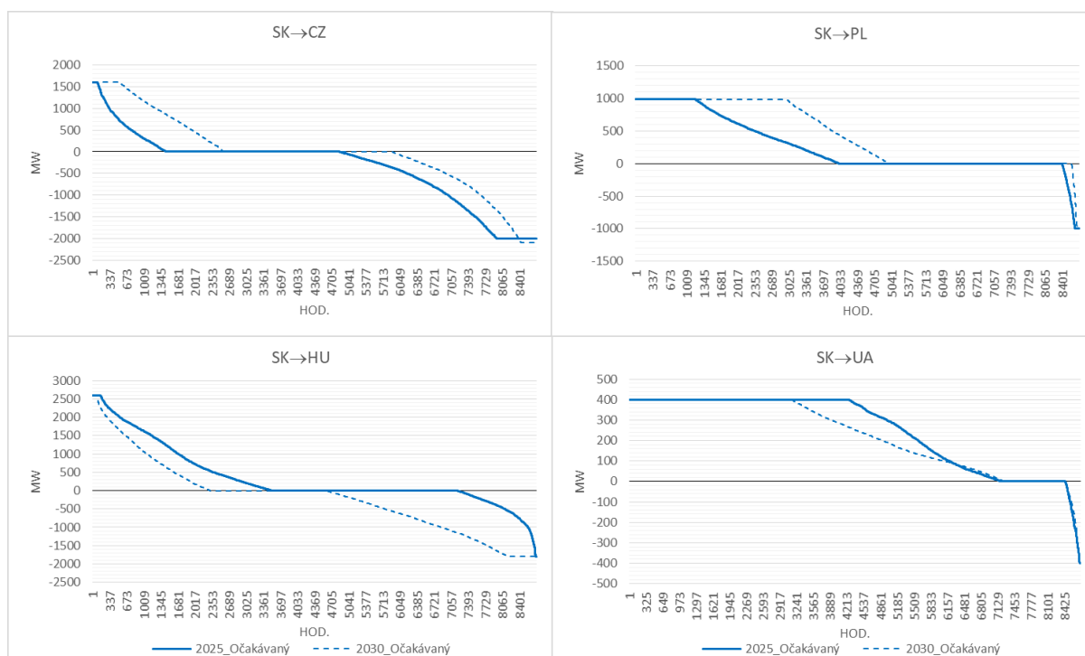
Obrázok č. 5.3.1_3 Predpokladané využitie NTC na jednotlivých cezhraničných profiloch pre očakávaný scenár v časových horizontoch 2025 a 2030 (pozn. kladné hodnoty znamenajú export)
