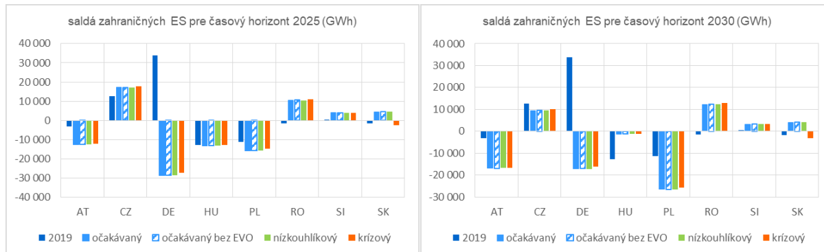
Obrázok č. 5.3.1_1 Saldá zahraničných ES pre časové horizonty 2025 a 2030 a rok 2019
