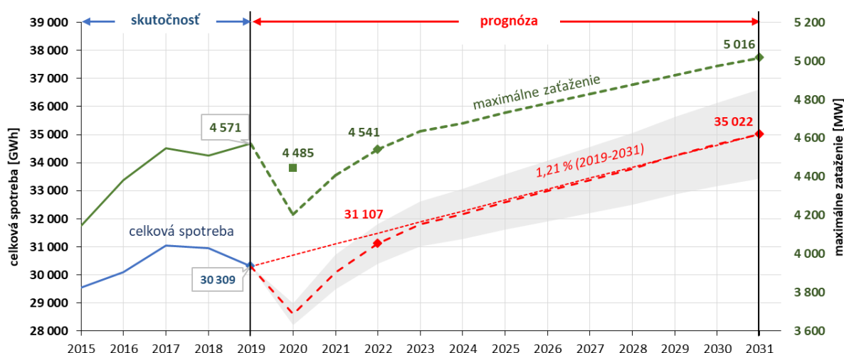
Obrázok č. 4.1.1_1 Predpokladaný vývoj spotreby elektriny a maximálneho zaťaženia v ES SR
