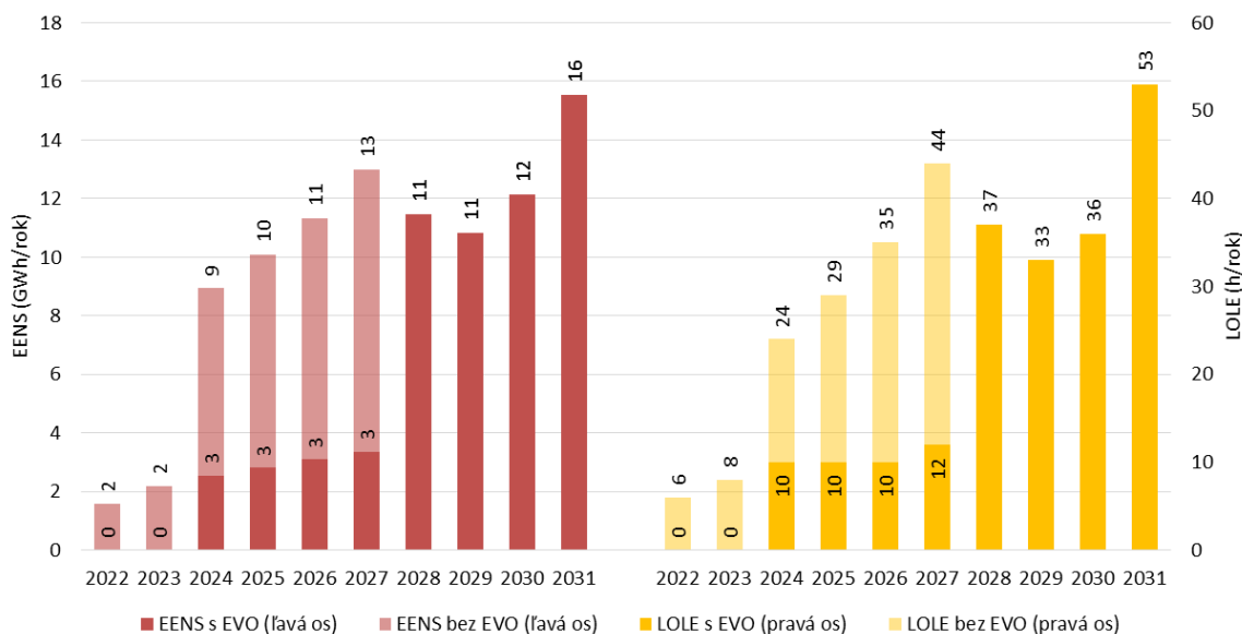
Obrázok č. 5.1_7 Ročné vyhodnotenie nedodanej energie – očakávaný scenár
