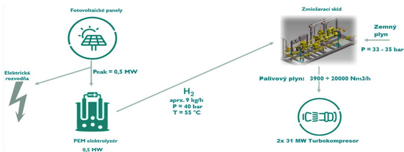
Obrázok č. 5 - schéma Green H2 na KS01
