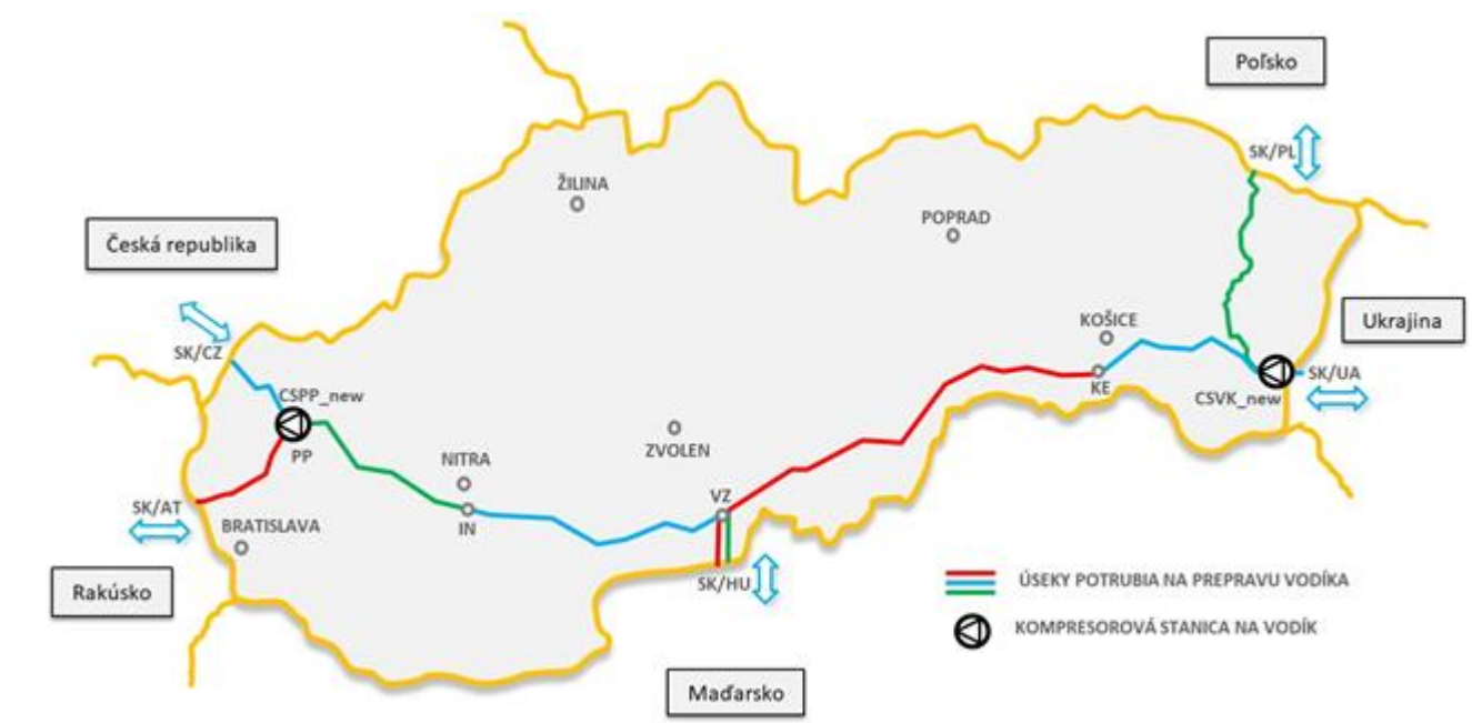
Obrázok č. 7 - Situačné znázornenie projektov
