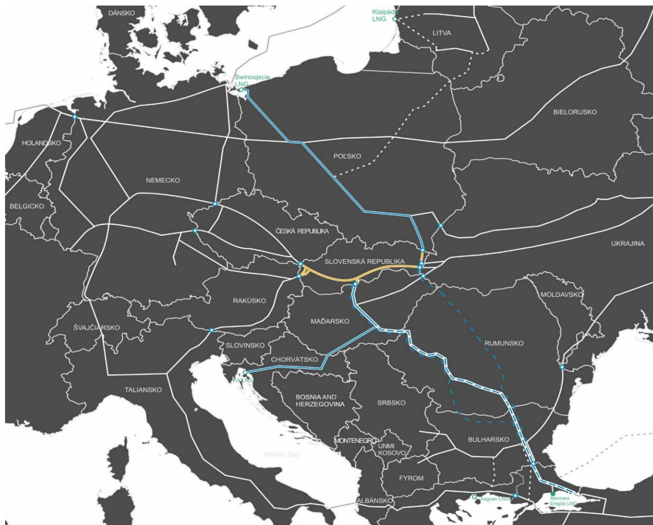
Obrázok č. 4 - Analyzované trasy plynovodu Eastring
