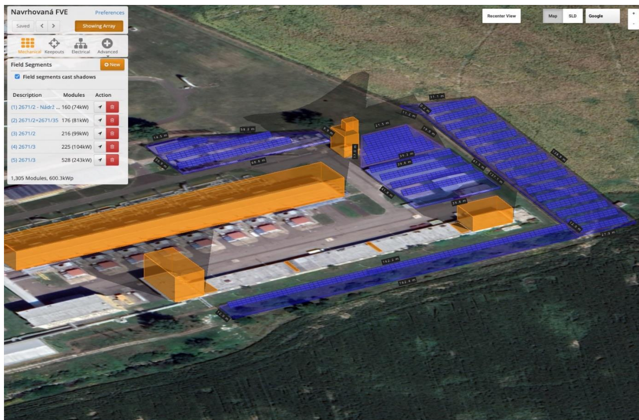
Obrázok č.6 – Predpokladané umiestnenie FV elektrárne na KS Veľké Kapušany
